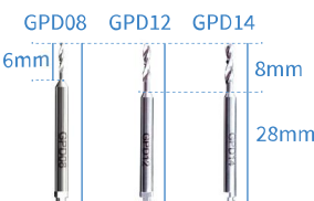
Guide drill 定位钻
