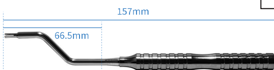
BTA03 膜钉持钉器 (Tack holder)
